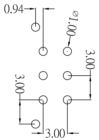
P.C.B. LAYOUT
