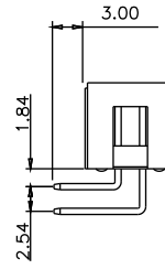
P/N:2316R-XXG
